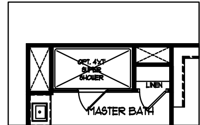
OPTIONAL SUPER SHOWER
